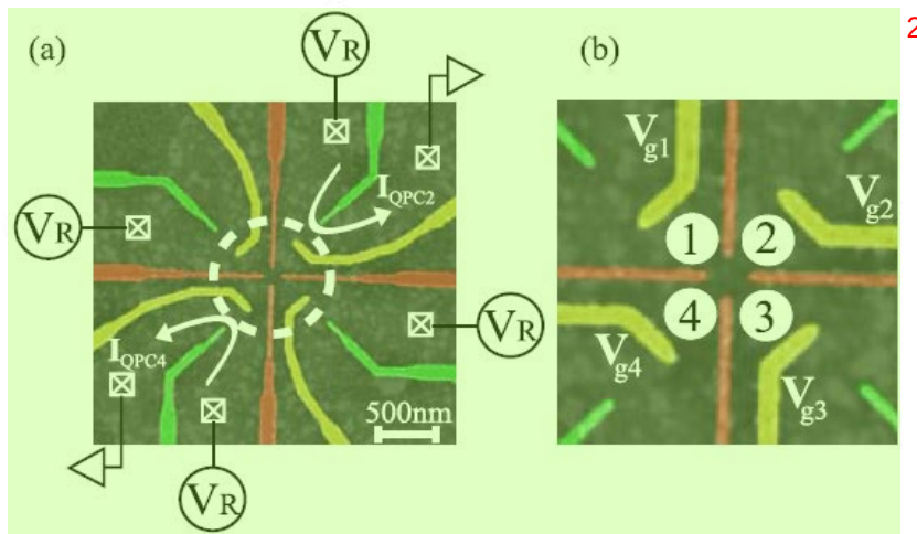
图 5.1 (a)四量子点对称结构设计样品扫描电镜结构图。(b)量子点区域放大结构图。图片引自文献[1]
