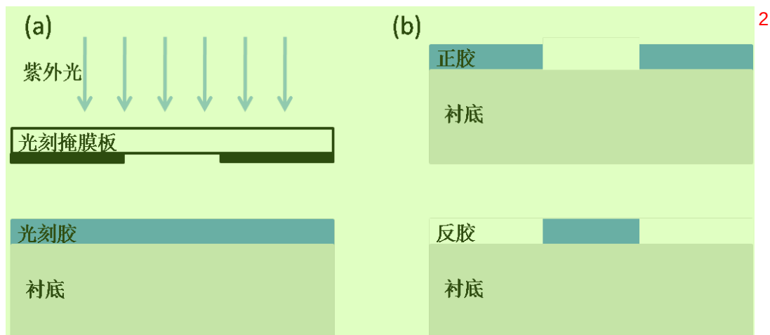
图 2.2 (a)光学曝光刻蚀示意图。(b)显影后正胶和反胶转移图形的示意图。
