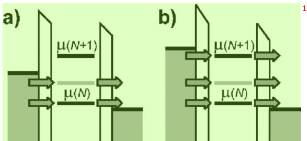
图 1.6 源漏电极在高偏压下隧穿电流情形。(a)第 N 个电子以及其激发态落入偏执电压区间，电子可以分别从第 N 个电子的基态和激发态这两条路径隧穿。(b)偏压过大时第 N+1 个电子也落入偏执电压区间。图片引自文献[31]
