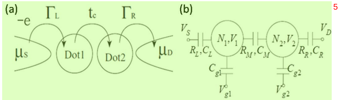
图 1.8 (a)串联双量子点耦合示意图 (b)串联双量子点等效电路图。图片引自文献[34] 6
