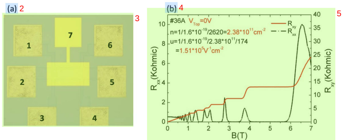
图 2.15 (a)Hall Bar 样品结构图。(b)测量的量子霍尔效应图。 6
