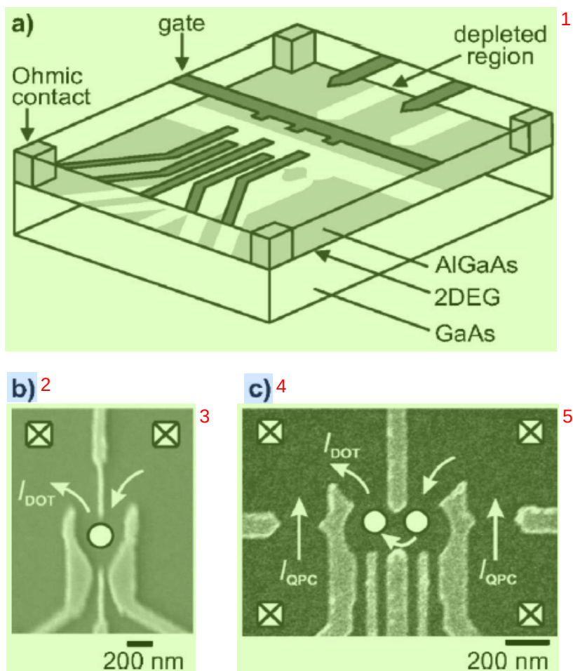
图 1.3 (a) 横向量子点结构示意图。在有二维电子气的 GaAs 通过表面门电极上施加电压来排挤下面电子，将中间电子约束。(b)-(c) 扫描电子显微镜下单量子点和串联双量子点结构。(c)中两侧为量子点接触结构(QPC)。图片引自文献[31]。
