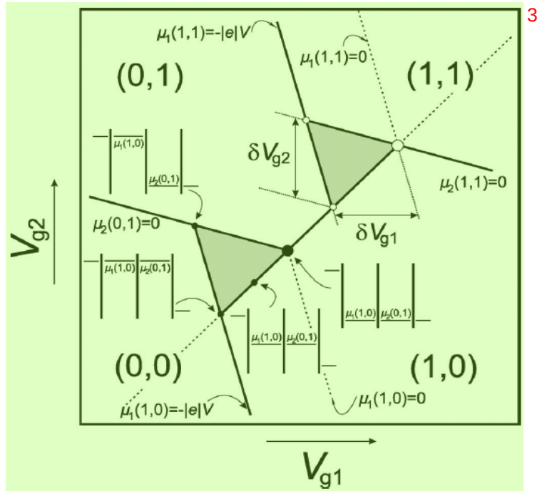
图 1.12 在源漏电极有偏执电压 V 的条件下的蜂窝图，三相点因为偏执电压而展成了偏压三角形。图中画出了偏压三角形每条边所对应的量子点中电化学势与源漏费米面的关系。图片引自文献[31] 4
