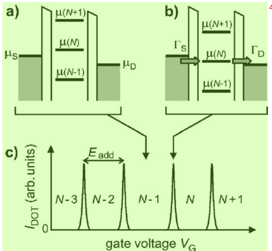
图 1.5 量子点中能级对应的电势示意图和库伦振荡示意图。(a)没有能级落入源漏偏压窗口中，没有电流通过，形成库伦阻塞。(b)电势 \mu(N) 刚好处在偏压窗口，发生电子隧穿，隧穿电流的大小取决于量子点与源漏之间的隧穿几率 \Gamma 。(c)量子点电流随栅极门电压调节的变化，即为库伦振荡。图片引自文献[31] 5
