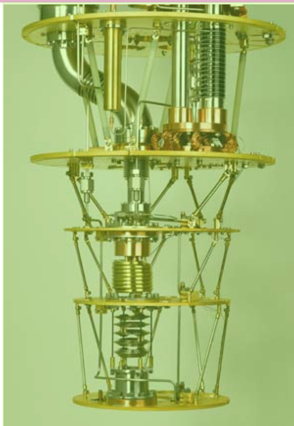
图 2.13 Triton 系统内部结构图。 4
