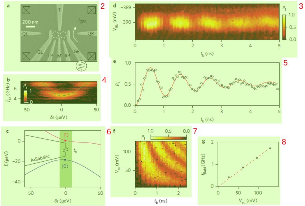
图 3.7 Si/SiGe 电荷量子点的拉比振荡。(a)样品扫描电镜图片。(b)量子点能级随微波 9 频谱的变化图。(c)施加微波波形示意图。(d)微波驱动下的拉比振荡。(e)提取出的振荡随时间数据，振荡周期为 1GHz。(f)(g)不同微波振幅驱动下振荡频率的变化关系。图片引自文献 [12]。
