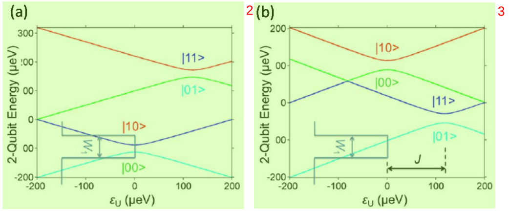
图 4.6 双电荷量子比特中计算的能级结构。(a)下面量子比特处于 |0\rangle 态时, 上面量子点的平衡点在 \varepsilon_U = 0 处。(b) 下面量子比特处于 |1\rangle 态时, 上面量子点的平衡点在 \varepsilon_U = J 处。可以看到下面量子点的状态对上面量子点的平衡点的影响程度为 J 。图片引自文献[10]
