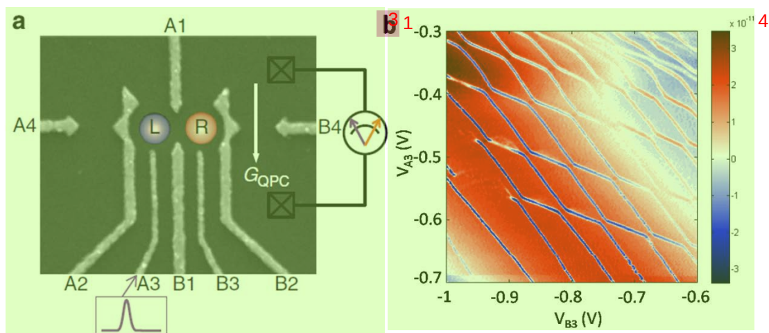
图 3.1 (a)扫描电镜下双量子点样品结构图。图片引自文献[9](b)测量的双量子点样品蜂窝图。 5
