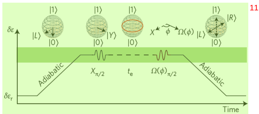
图 3.8 Ramsey 操作波形示意图。图片引自文献[12]。 12
