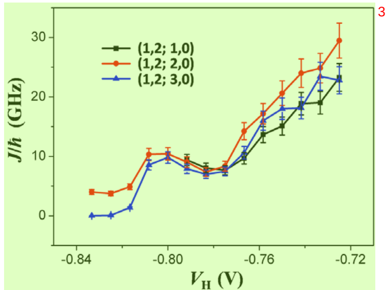
图 4.4 耦合能量 J 随水平门电极电压 V_H 的变化曲线。 J 值的测量选取的电子为 (M_U, N_U; M_L-1, N_L+1) 和 (M_U-1, N_U+1; M_L, N_L) , 其中 (M_U, N_U) 固定在电子数为 (1, 2)处, (M_L, N_L) 变化从(1, 0)到(2, 0)再到(3, 0),分别对应图中黑色、红色和蓝色的线。图片引自文献[9]
