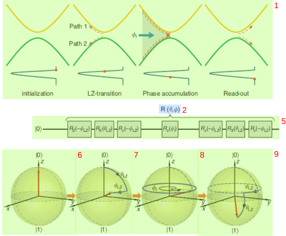
图 3.6 在布洛赫球面上演示 LZS 四步演化过程。图片引自文献[9]
