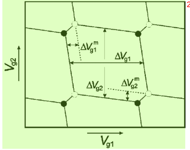
图 1.10 双量子点系统蜂窝图原胞结构, 图中黑白色点为三相点, 双量子点发生共振隧穿, \Delta V_{g1} 和 \Delta V_{g2} 为每个量子点的充电能, \Delta V_{g1}^m , \Delta V_{g2}^m 为每个量子点的相互耦合充电电压。图片引自文献[34]
