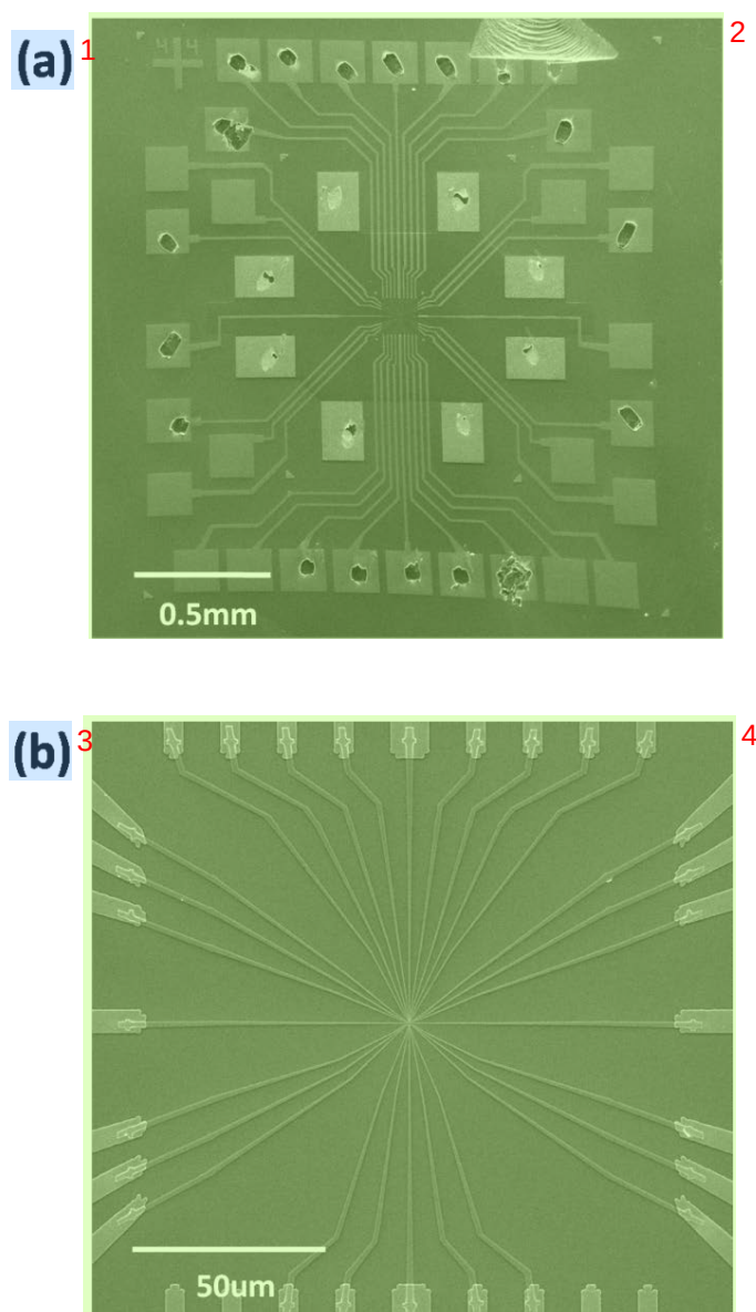
图 2.12 使用扫描电镜拍摄的样品结构图。(a)测量过的样品图像。(b)内部使用电子束曝光的小结构。
