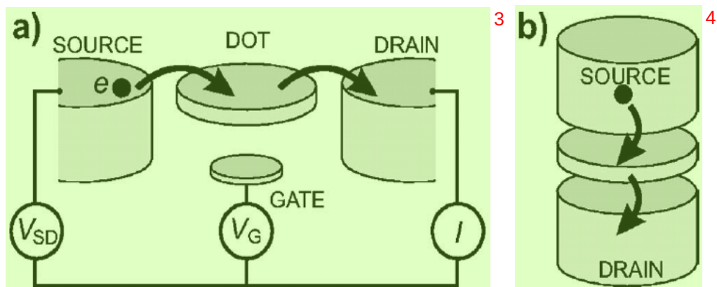
图 1.1 横向和纵向两种不同量子点的示意图，电子通过源极(Source)流经量子点(圆盘形式)到漏记(Drain),通过门电压 V_G 可以对量子点中的电子数据进行调节。(a)横向分布的量子点结构示意图。(b)纵向分布量子点示意图。图片引自文献[31]。
