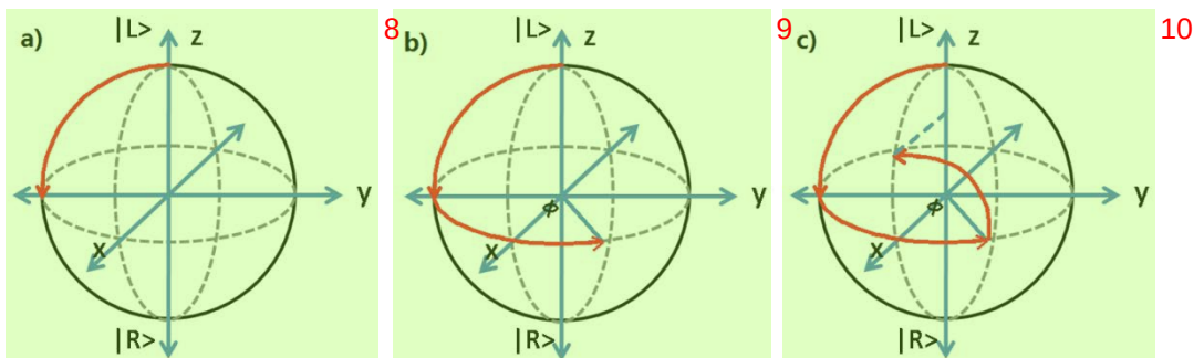
图 3.4 在布洛赫球面演示二能级体系随脉冲变化。(a)脉冲使得从远离平衡点到刚好到 11
