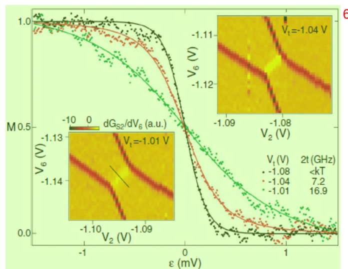
图 3.2 双量子点中电子在平衡点附近的占据状态变化。图片引自文献[10] 7
