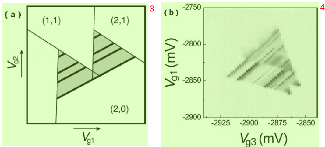
图 1.13 偏压三角形在源漏电极高偏执电压下出现的激发态能级。(a)偏压三角形在高偏执电压下出现的激发态能级示意图。(b)实验中通过测量量子点输运电流所看到的偏压三角形中的激发态能级。通过施加反向的偏压可以使偏压三角形反转。的图片引自文献[34]
