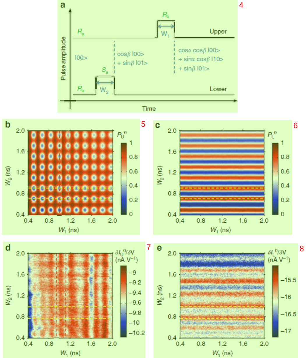
图 4.8 (a)上下两个电荷量子比特操作波形示意图。(b)(c)分别代表理论模拟计算下 P_U^0 和 P_L^0 在脉冲驱动下的几率变化图像。(d)(e)实验测量到分别流经上下量子比特探测的 QPC 通道的电流变化。图片引自文献[10]
